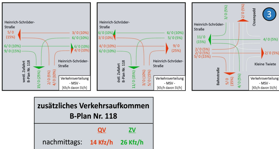
Abbildung 3.5: Verteilung des zusätzlichen Verkehrsaufkommens, H.-S.-Straße – MSV
