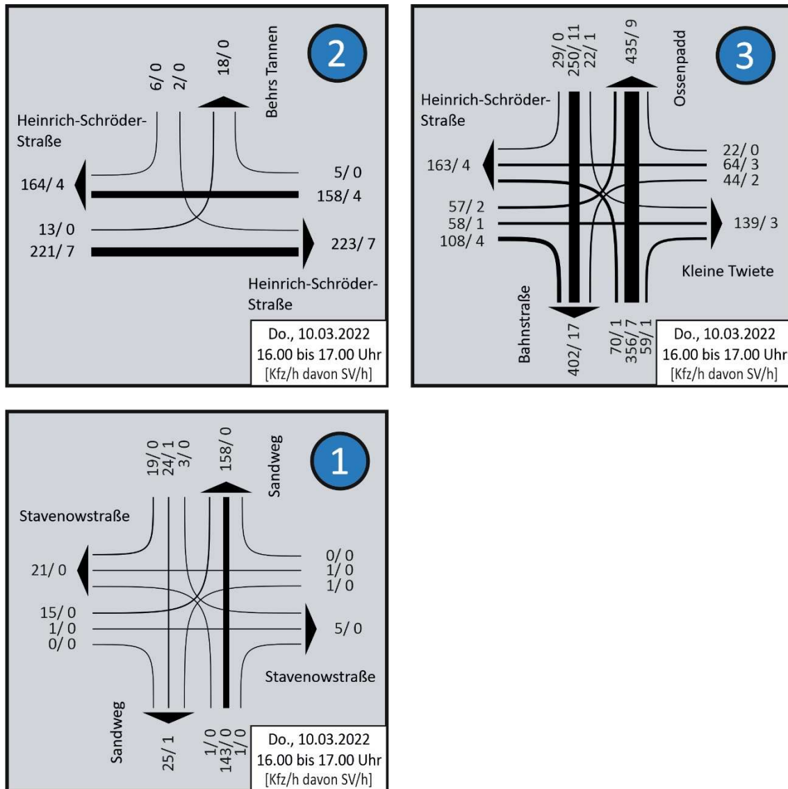
Abbildung 2.3: Analyse 2022 – Spitzenstunde, nachmittags
