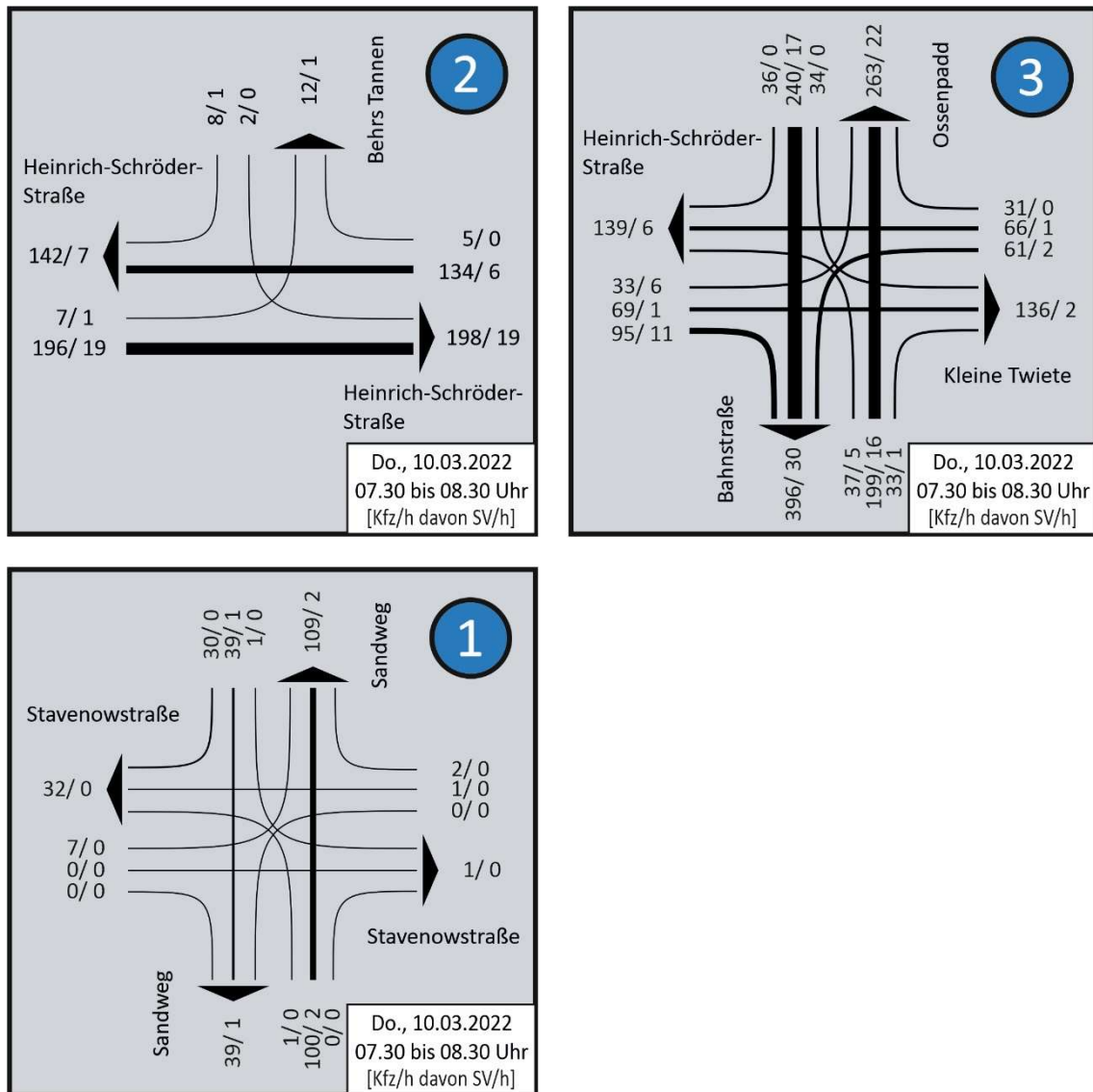
Abbildung 2.2: Analyse 2022 – Spitzenstunde, morgens
