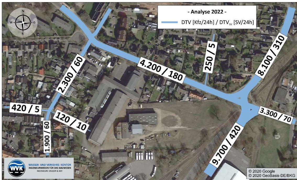
Abbildung 2.4: Analyse 2022 – DTV, DTV sv
