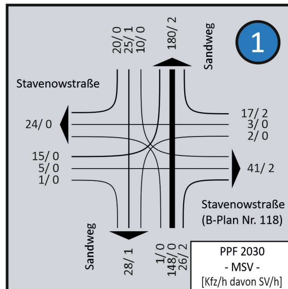
Abbildung 3.6: Prognose-Planfall 2030, Sandweg– MSV
